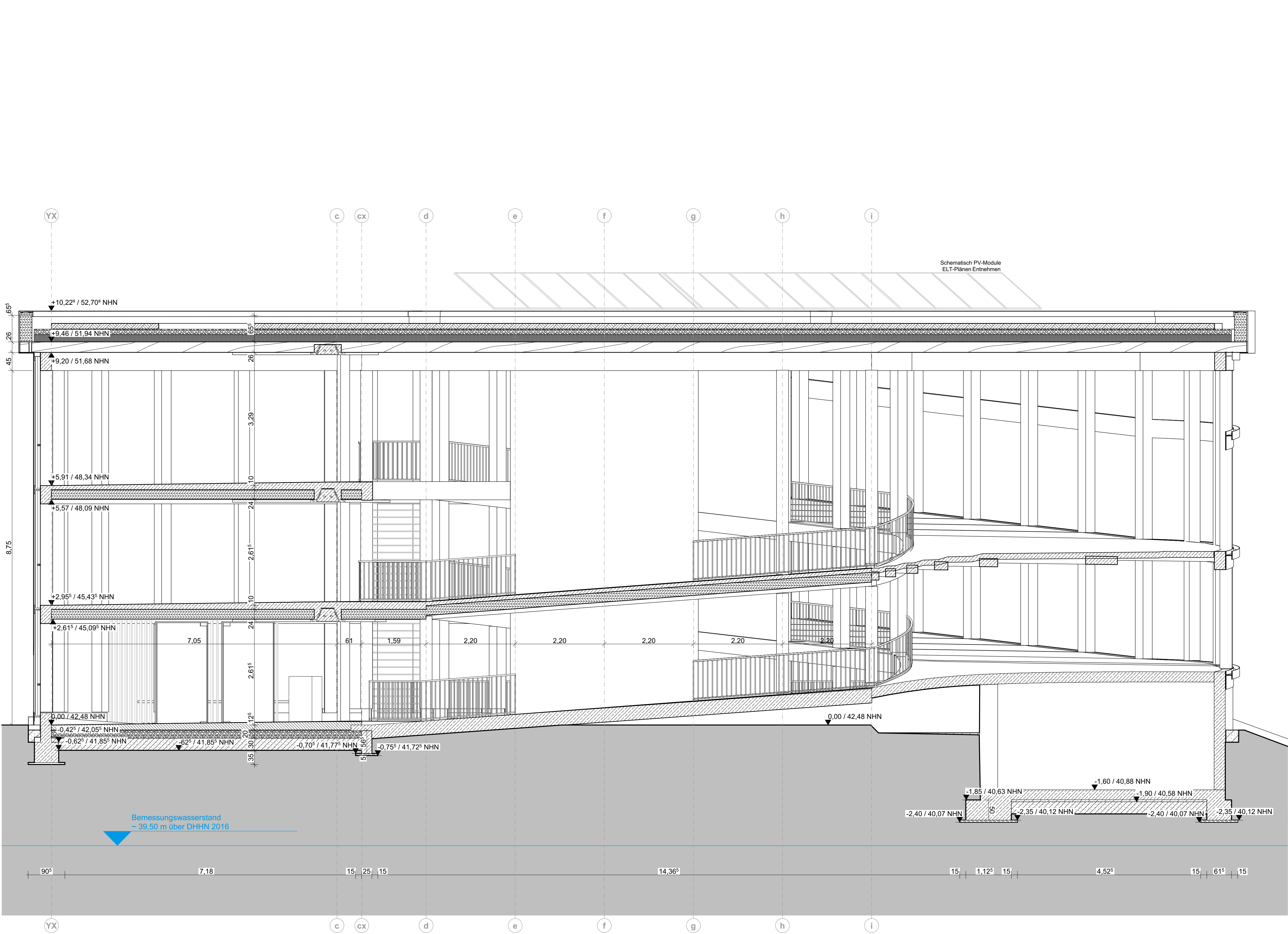
Schnitt West-Ost
